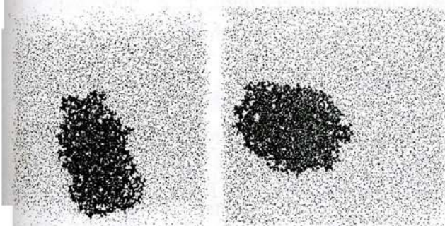
Рис. 2. Структура компьютерной модели ПВС в водном растворе: а – при t = 0 нс; б – t = 30 нс
