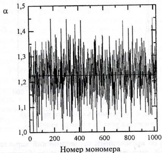
Рис. 6. Зависимость угла \alpha от номера мономера
