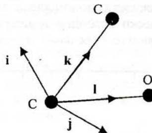
Рис. 3. Схема построения ортонормированного базиса в мономере
