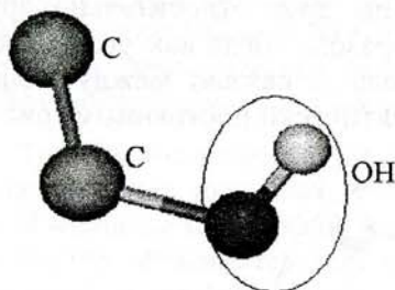
Рис. 1. Мономерное звено полимера ПВС
