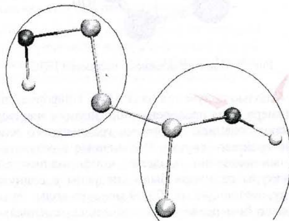
Рис. 7. Два мономерных звена полимера ПВС
